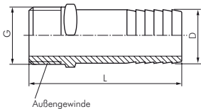
Außengewinde
