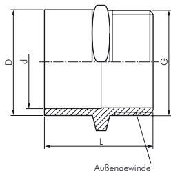
Außengewinde
