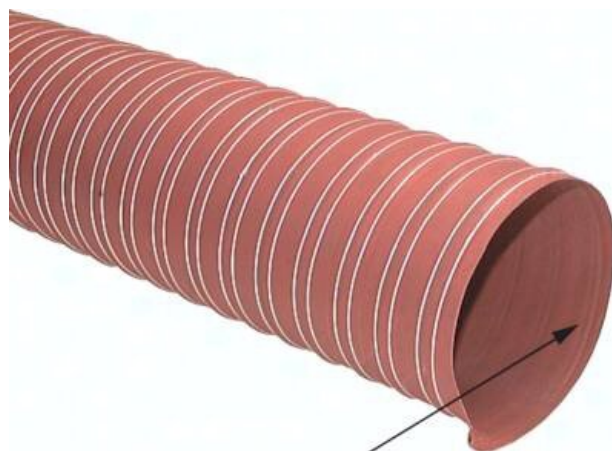
eingewähte Drahtspirale
